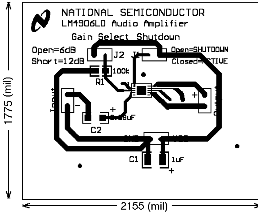
Top Layer
